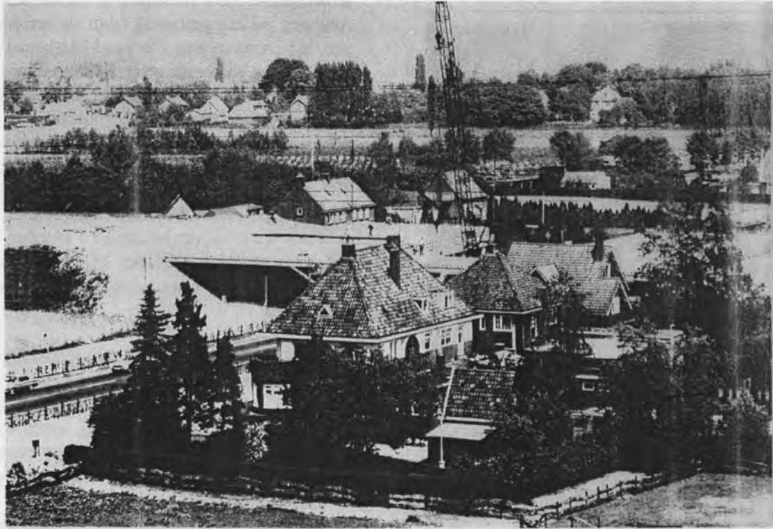
Bouw van het viaduct aan de Graafsebaan te Hintham. Rechts zien we de panden Hintham 123-125-127-129.
