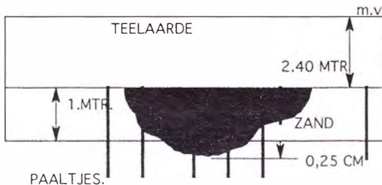
PROFIEL WATERPUT NOORDELIJKE ZIJDE
