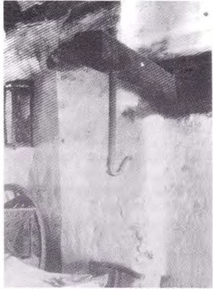
Gezicht vanaf de voorstal op de achterzijde van de brandmuur, met de door de sleuf naast de deur stekende arm van de draaiboom (foto: SHBO).
